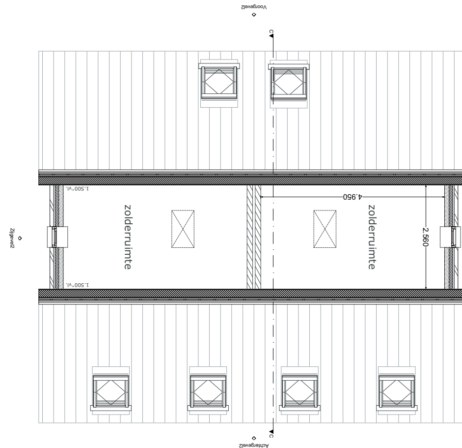
2 e verdieping
